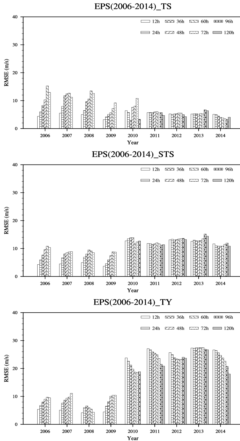
그림 3.7.12 앙상블예측시스템(EPSS)의 태풍 최대풍속 모의 성능 변화(2006~2010년(T213L40), 2011년 이후(UM N320L70))
