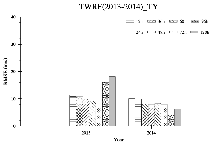
그림 3.7.13 태풍예측시스템(TWRF)의 최대풍속 모의 성능 변화
