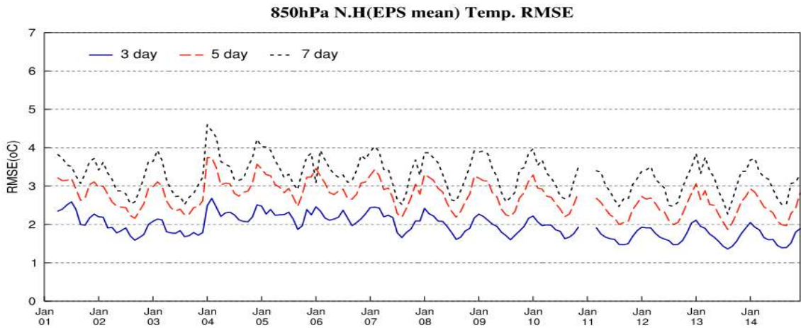
그림 3.4.4 EPSG 북반구 850hPa 기온의 예측 시간별 월평균 RMSE
