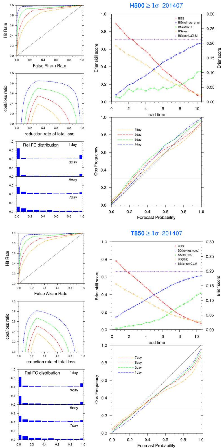
그림 3.4.13 2014년 7월 EPSG 북반구 500 hPa 고도(상)와 850hPa 기온(하)의 +1 표준편차에 대한 확률예측 성능 (왼쪽 상단부터 ROC curve, Economic Value, Rank histogram, 오른쪽 상단부터 Brier Score, Reliability Table)
