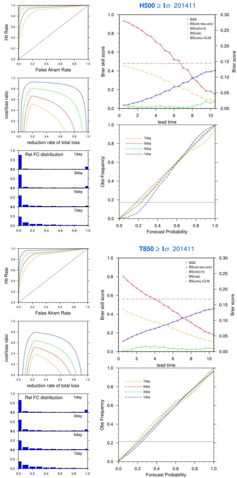
그림 3.4.17 2014년 11월 EPSG 북반구 500 hPa 고도(상)와 850hPa 기온(하)의 +1 표준편차에 대한 확률예측 성능 (왼쪽 상단부터 ROC curve, Economic Value, Rank histogram, 오른쪽 상단부터 Brier Score, Reliability Table)
