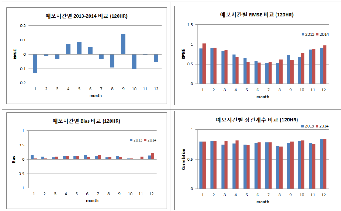
그림 3.6.9 GWW3 +120H 예보장에 대한 전년 대비 성능 비교. BIAS, RMSE, Correlation
