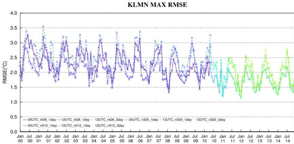
그림 3.5.1 KLMN 최고기온 월별 RMSE 성능 변화
