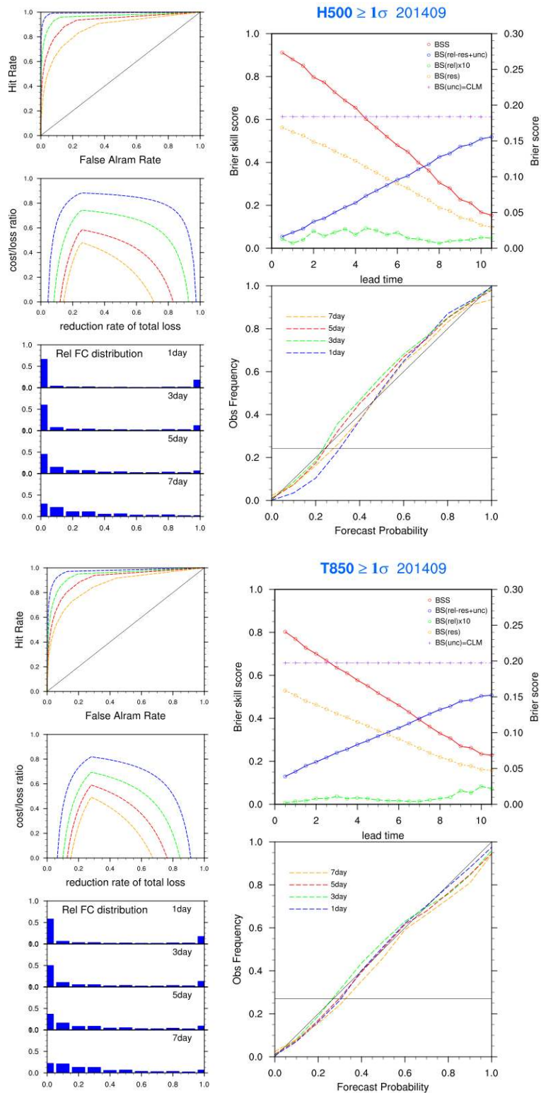
그림 3.4.15 2014년 9월 EPSG 북반구 500 hPa 고도(상)와 850hPa 기온(하)의 +1 표준편차에 대한 확률예측 성능 (왼쪽 상단부터 ROC curve, Economic Value, Rank histogram, 오른쪽 상단부터 Brier Score, Reliability Table)
