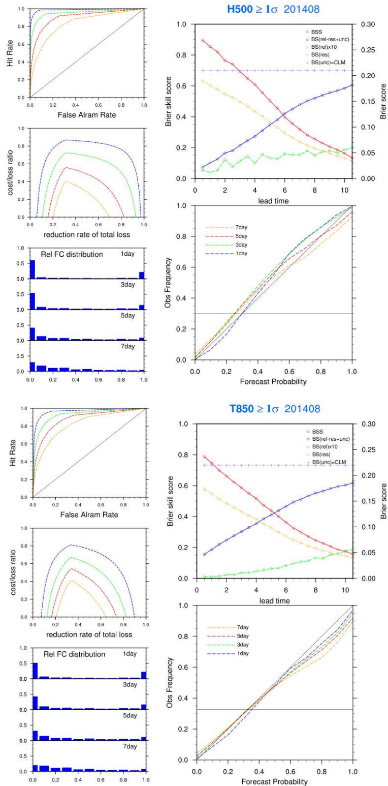
그림 3.4.14 2014년 8월 EPSG 북반구 500 hPa 고도(상)와 850hPa 기온(하)의 +1 표준편차에 대한 확률예측 성능 (왼쪽 상단부터 ROC curve, Economic Value, Rank histogram, 오른쪽 상단부터 Brier Score, Reliability Table)
