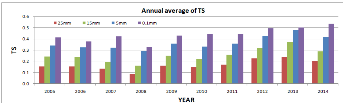
그림 2.9 2005년 이후 지역예측시스템 강수 예측에 대한 성공임계지수의 년 평균 변화
