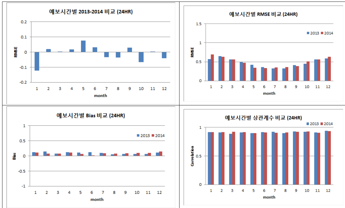
그림 3.6.5 GWW3 +24H 예보장에 대한 전년 대비 성능 비교. BIAS, RMSE, Correlation
