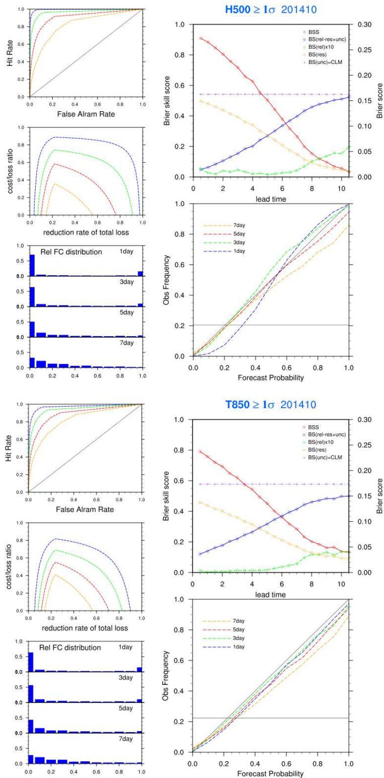
그림 3.4.16 2014년 10월 EPSG 북반구 500 hPa 고도(상)와 850hPa 기온(하)의 +1 표준편차에 대한 확률예측 성능 (왼쪽 상단부터 ROC curve, Economic Value, Rank histogram, 오른쪽 상단부터 Brier Score, Reliability Table)
