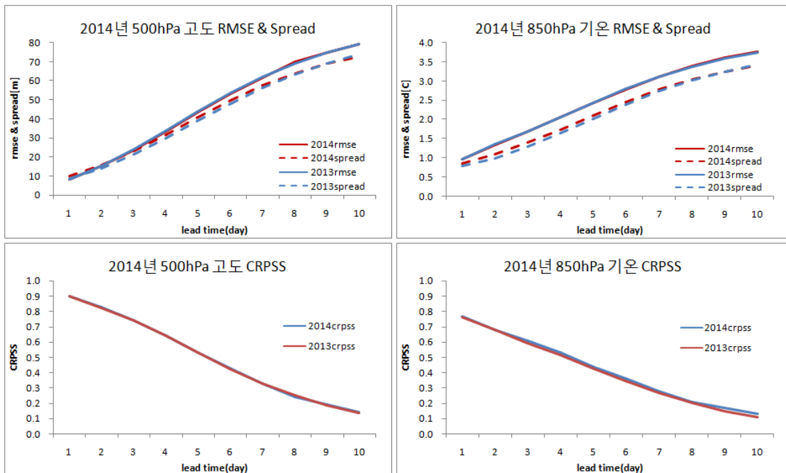
그림 2.11 2013년 및 2014년 EPSG 북반구 평균 RMSE/Spread와 CRPSS
