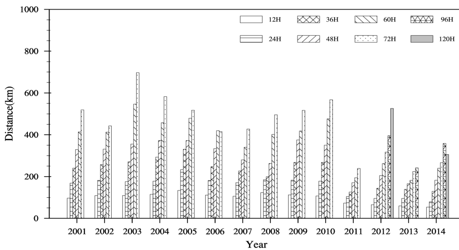
그림 3.7.3 앙상블예측시스템(EPSP)의 태풍진로오차 성능 변화(2001~2005년(T106L30), 2006~2010년(T213L40), 2011년 이후(UM N320L70))
