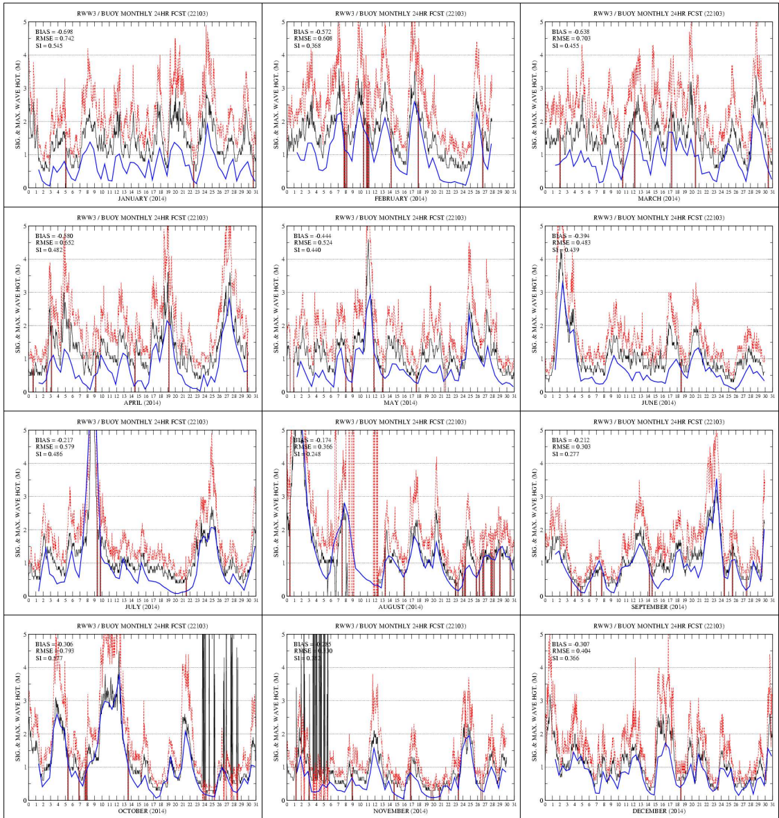
그림 3.6.12 거문도 부이 관측(검은색 실선)과 RWW3 +24H 예측 유의파고(파란색 실선) 시계열 (2014년 1월~12월). 붉은색 점선은 최대 파고
