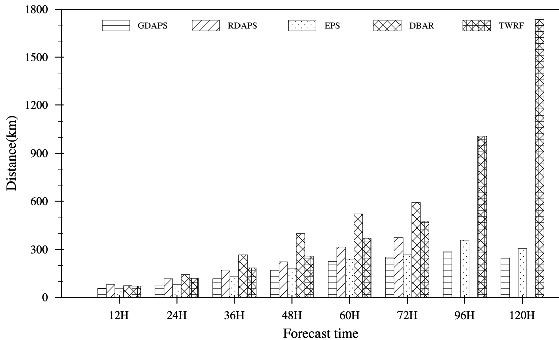
그림 3.7.6 2014년 모델별 태풍 진로의 단순거리오차(Direct Position Error)
