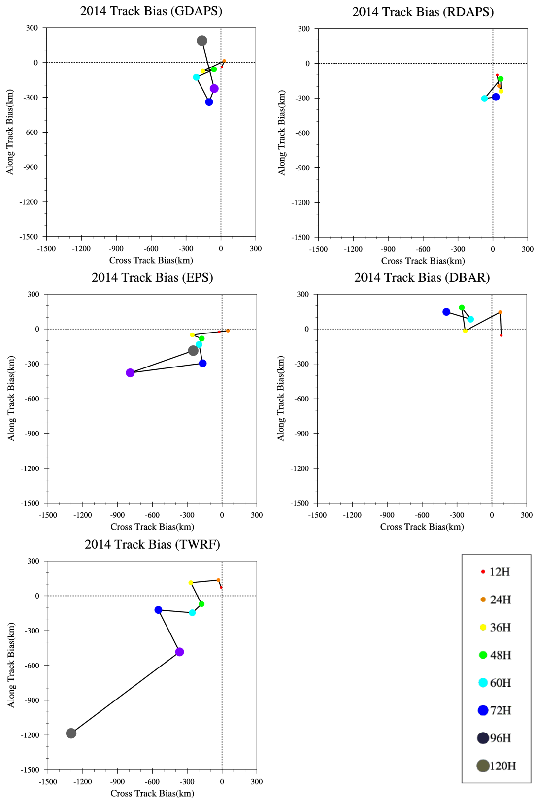
그림 3.7.9 2014년 모델별 태풍 진로의 Track Bias (Median)
