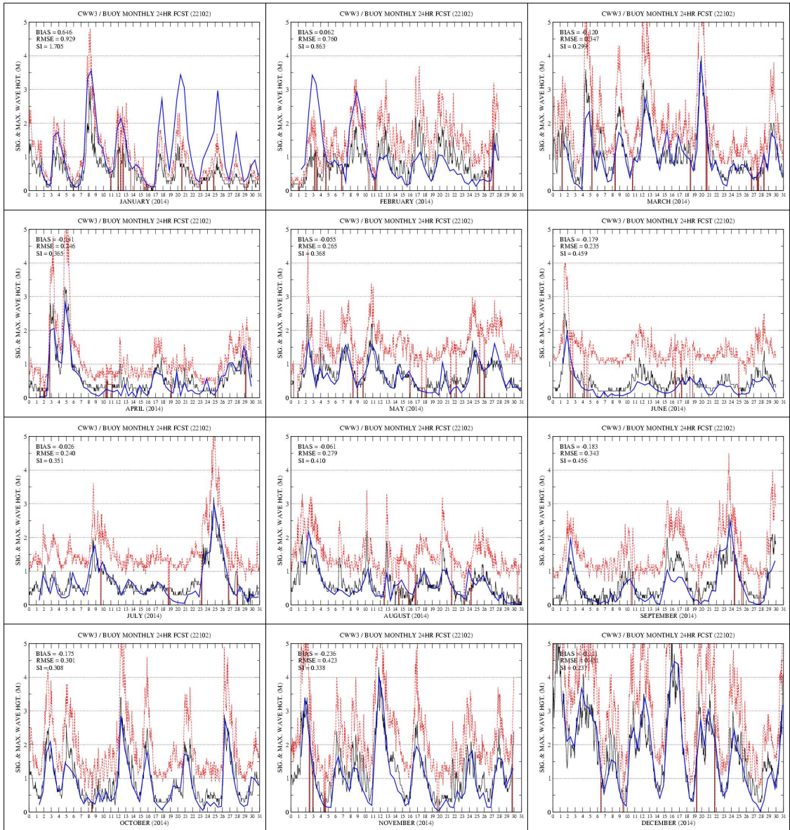
그림 3.6.19 칠발도 부이 관측(검은색 실선)과 CWW3 +24H 예측 유의파고(파란색 실선) 시계열 (2014년 1월~12월). 붉은색 점선은 최대 파고
