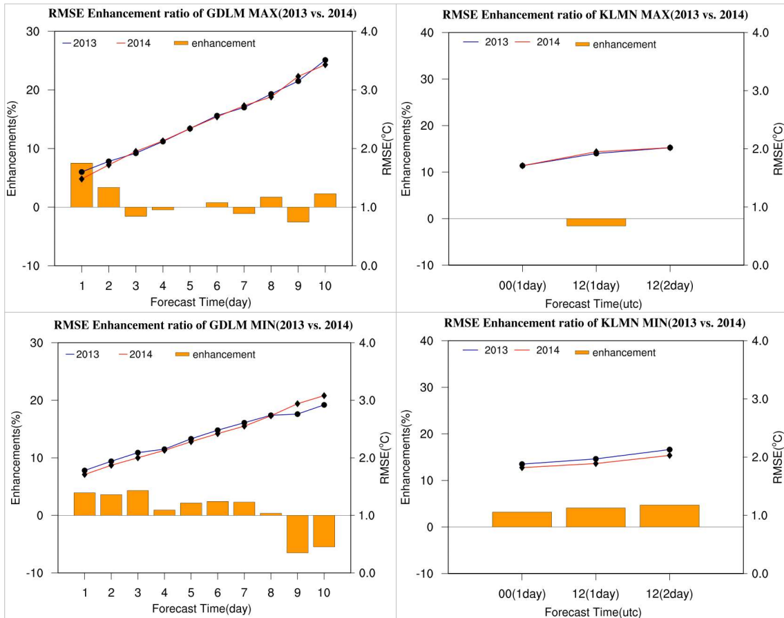
그림 2.12 통계예측시스템 GDLM(좌) 및 KLMN(우) 2013년 대비 2014년 개선 정도
