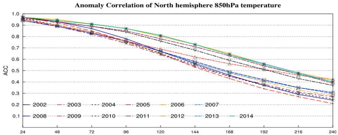
그림 2.3 전지구예측시스템(GDAPS) 북반구 850hPa 기온 분석검증 이상상관 계수 예보시간별, 년별 변화
