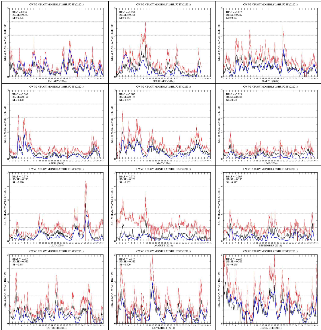
그림 3.6.18 덕적도 부이 관측(검은색 실선)과 CWW3 +24H 예측 유의파고(파란색 실선) 시계열 (2014년 1월~12월). 붉은색 점선은 최대 파고
