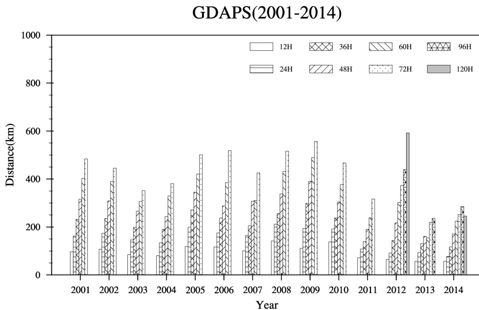
그림 3.7.1 전지구예측시스템 (GDAPS)의 태풍진로오차 성능 변화(2006년 이전(T213L30), 2006~2009년(T426L40), 2010년(UM N320L50), 2011년 이후(UM N512L70))
