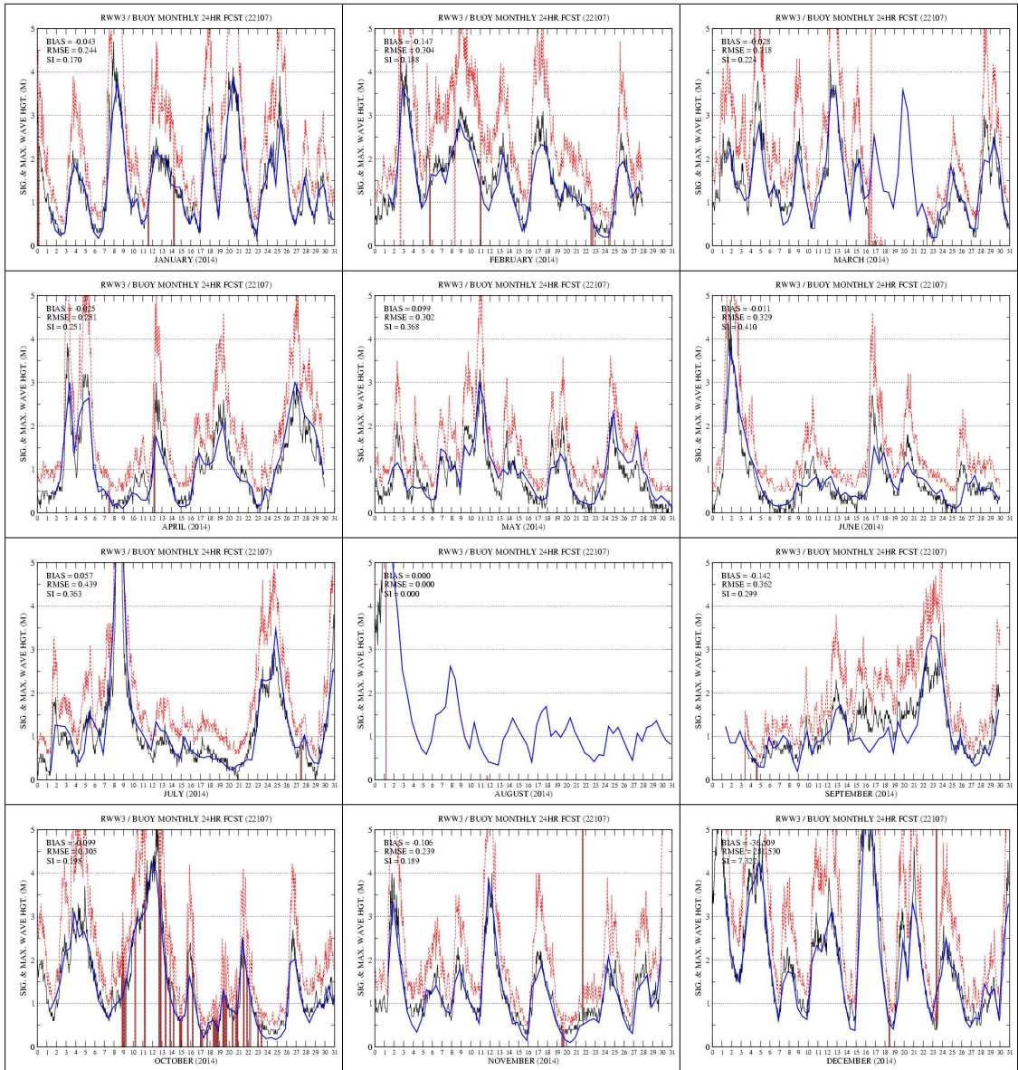
그림 3.6.16 마라도 부이 관측(검은색 실선)과 RWW3 +24H 예측 유의파고(파란색 실선) 시계열 (2014년 1월~12월). 붉은색 점선은 최대 파고
