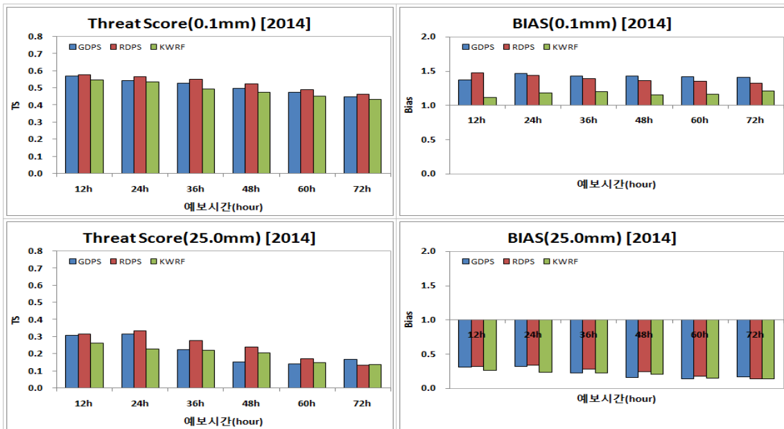
그림 2.8 예측시스템별 2014년 강수 검증(좌: TS, 우: BIAS)
