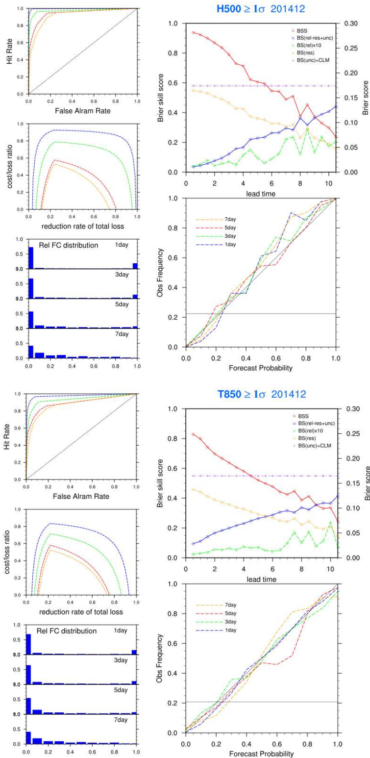
그림 3.4.18 2014년 12월 EPSG 북반구 500 hPa 고도(상)와 850hPa 기온(하)의 +1 표준편차에 대한 확률예측 성능 (왼쪽 상단부터 ROC curve, Economic Value, Rank histogram, 오른쪽 상단부터 Brier Score, Reliability Table)
