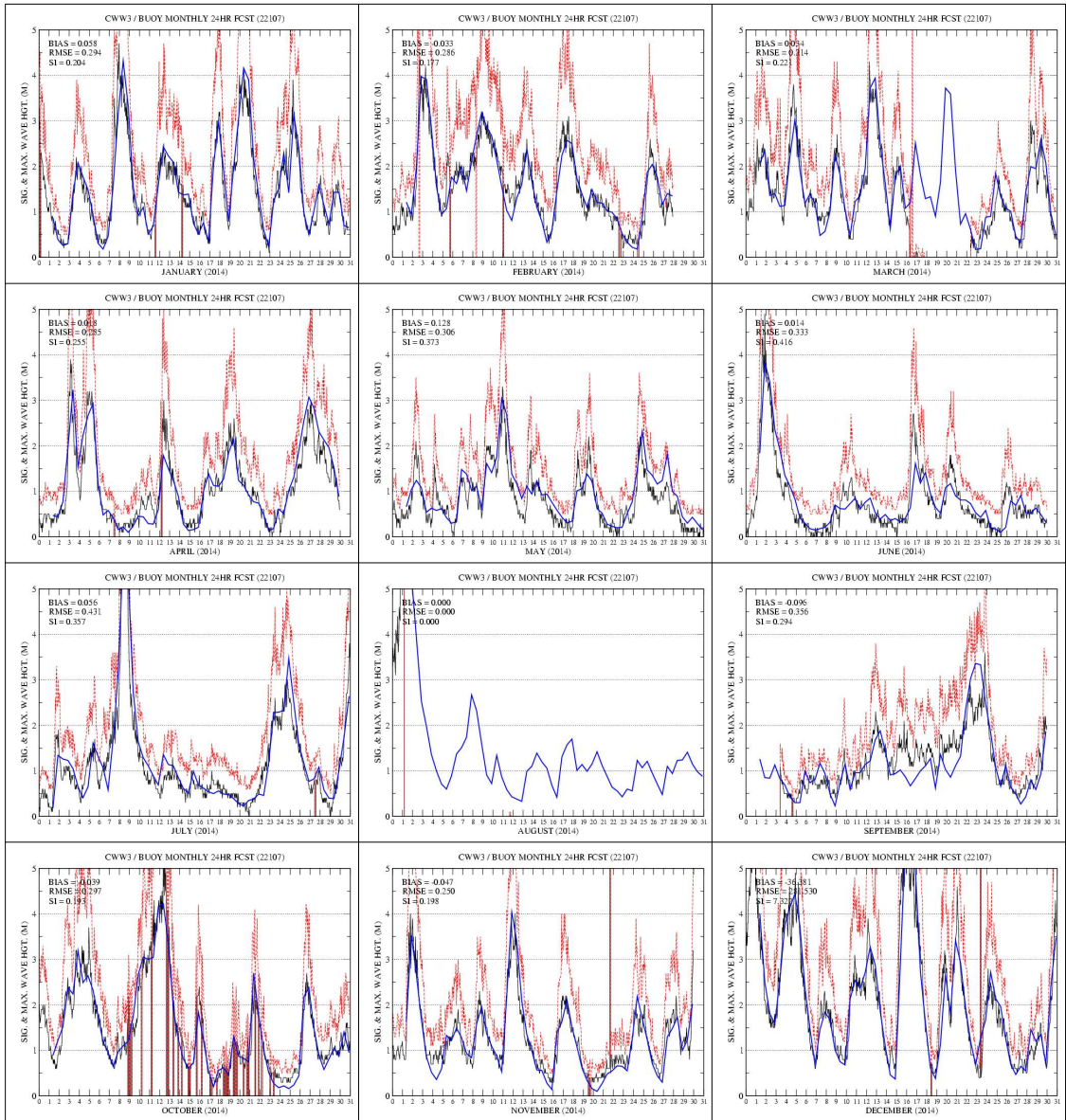
그림 3.6.24 마라도 부이 관측(검은색 실선)과 CWW3 +24H 예측 유의파고(파란색 실선) 시계열 (2014년 11월~12월). 붉은색 점선은 최대 파고
