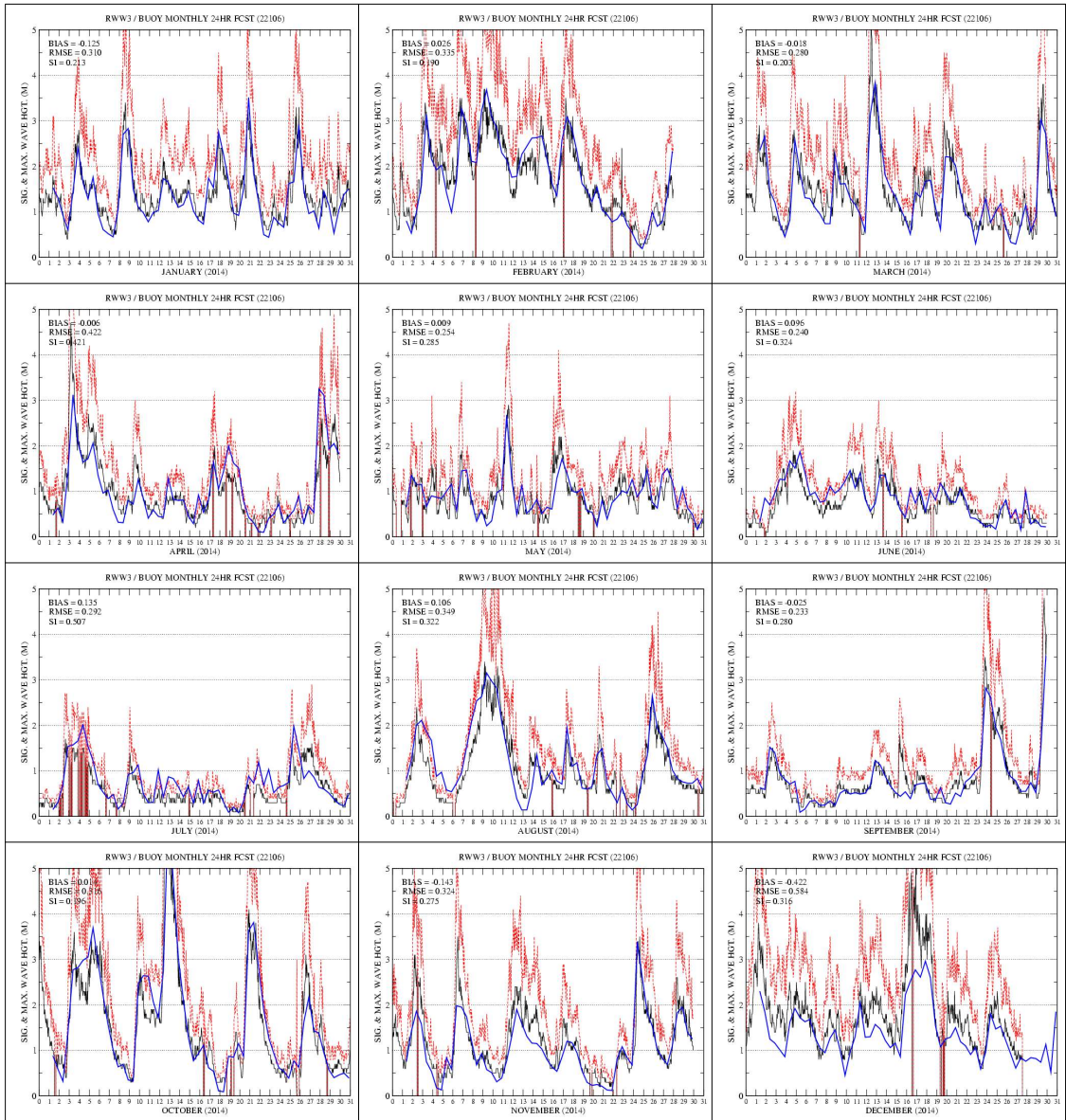
그림 3.6.15 포항 부이 관측(검은색 실선)과 RWW3 +24H 예측 유의파고(파란색 실선) 시계열 (2014년 1월~12월). 붉은색 점선은 최대 파고
