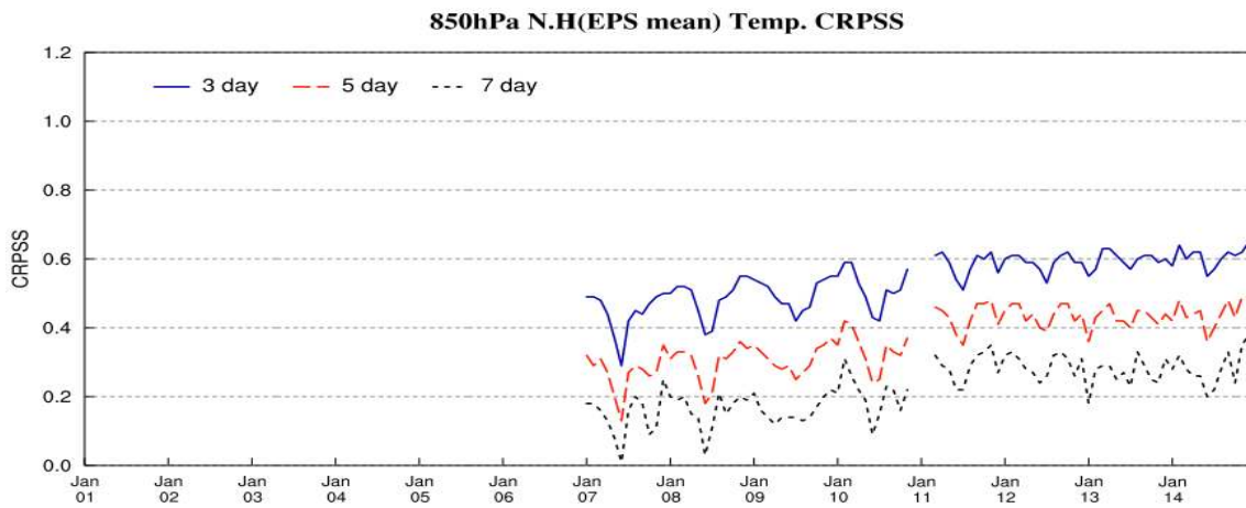
그림 3.4.6 EPSG 북반구 850hPa 기온의 예측 시간별 월평균 CRPSS
