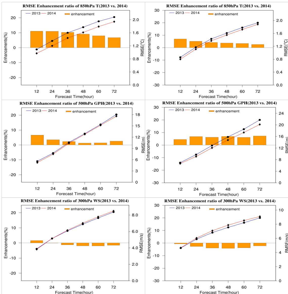
그림 2.7 지역예측시스템(UM 12km L70(좌)과 KWRF 10km L40(우)) 분석검증 RMSE 2013년 대비 2014년 개선 정도
