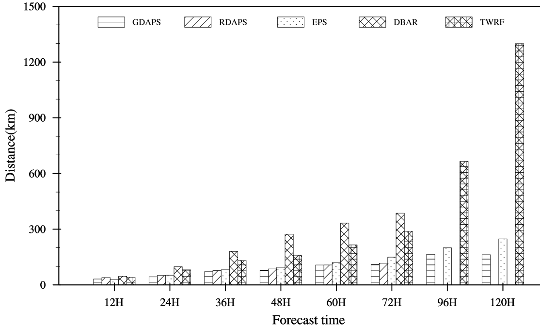
그림 3.7.8 2014년 모델별 태풍 진로의 방향오차(Cross Track Error)
