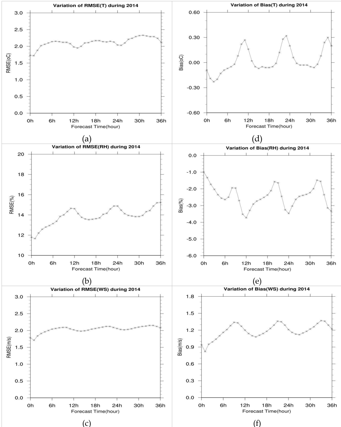
그림 3.3.1 LDAPS의 2014년 지상변수의 예보시간별 RMSE((a): 기온, (b): 상대습도, (c): 풍속) 및 Bias((d): 기온, (e): 상대습도, (f): 풍속)의 변화
