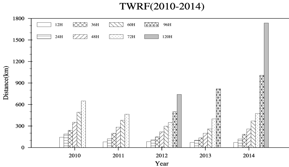
그림 3.7.5 태풍예측시스템(TWRF)의 태풍진로오차 성능 변화
