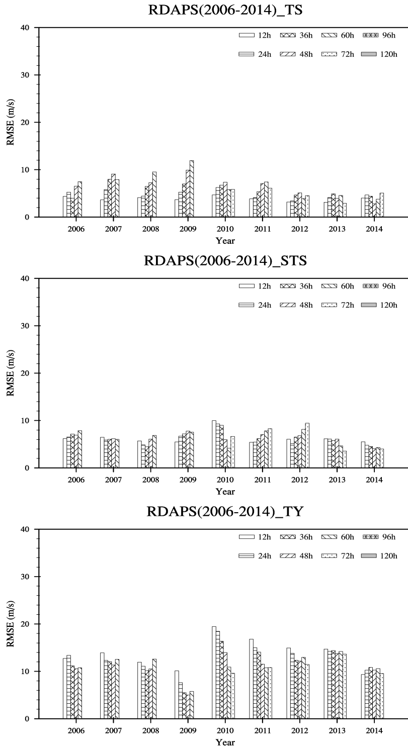
그림 3.7.11 지역예측시스템(RDAPS)의 태풍 최대풍속 모의 성능 변화(2009년 이전(MM5 30km), 2010년(UM 12km L38), 2011년 이후(UM 12km L70))
