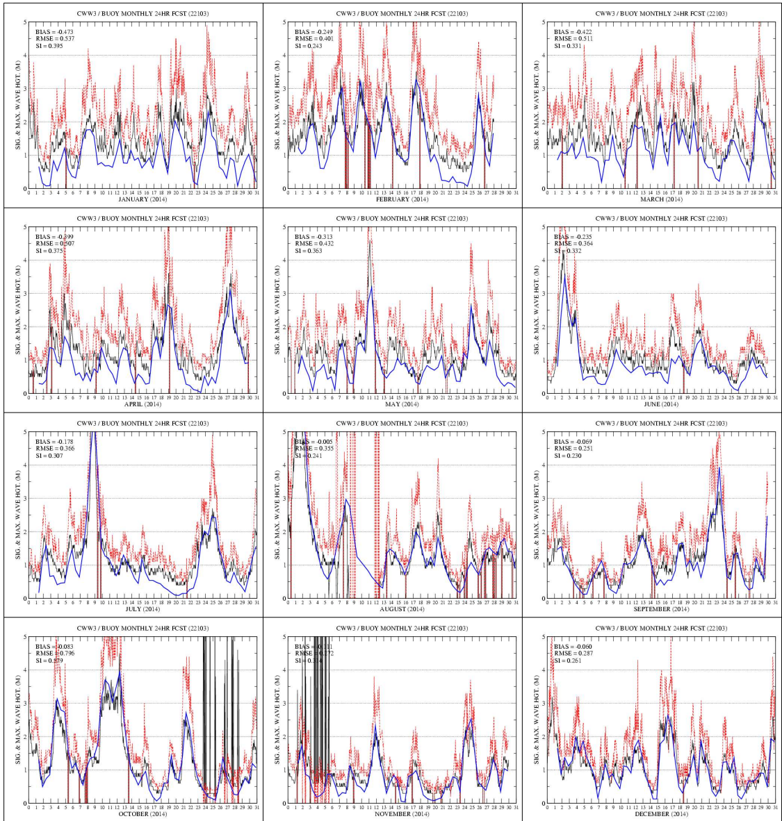
그림 3.6.20 거문도 부이 관측(검은색 실선)과 CWW3 +24H 예측 유의파고(파란색 실선) 시계열 (2014년 1월~12월). 붉은색 점선은 최대 파고
