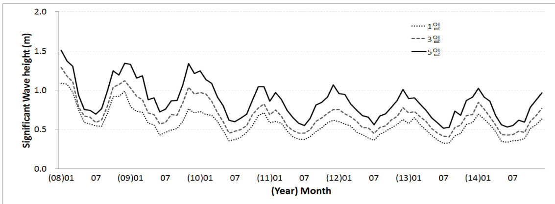
그림 3.6.2 전지구 파랑예측시스템(GWW3) 유의파고 부이검증 RMSE
