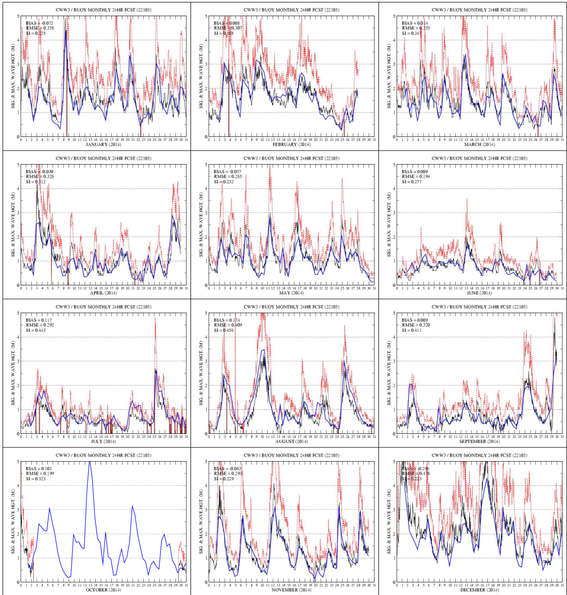
그림 3.6.22 동해 부이 관측(검은색 실선)과 CWW3 +24H 예측 유의파고(파란색 실선) 시계열 (2014년 1월~12월). 붉은색 점선은 최대 파고
