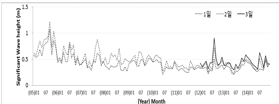
그림 3.6.3 지역 파랑예측시스템(RWW3) 유의파고 부이검증 RMSE
