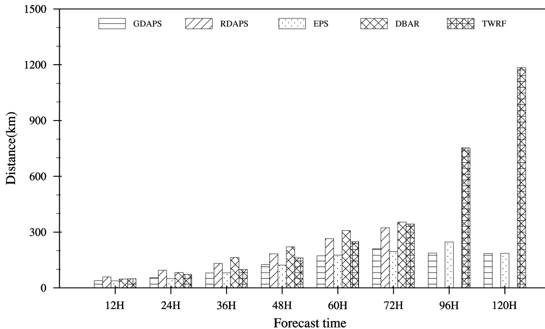
그림 3.7.7 2014년 모델별 태풍 진로의 이동속도오차(Along Track Error)
