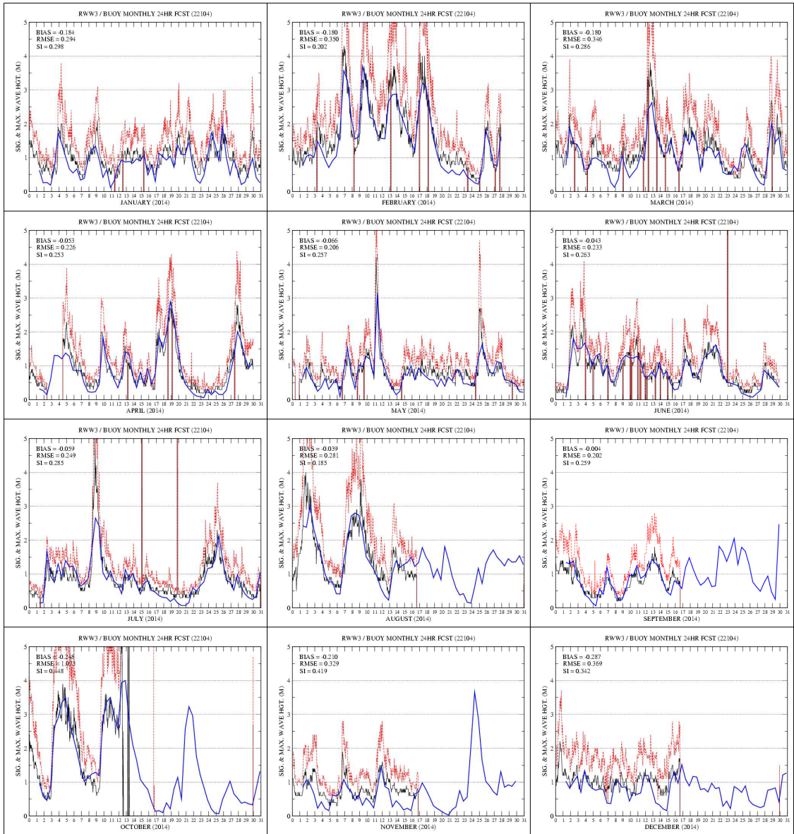
그림 3.6.13 거제도 부이 관측(검은색 실선)과 RWW3 +24H 예측 유의파고(파란색 실선) 시계열 (2014년 1월~12월). 붉은색 점선은 최대 파고
