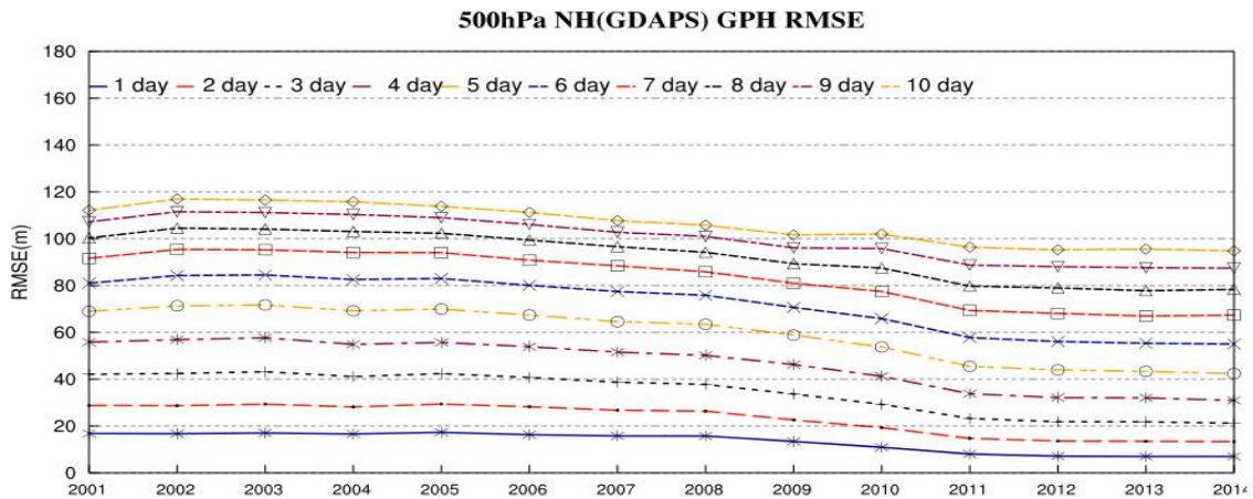
그림 2.2 전지구예측시스템(GDAPS) 북반구 분석검증 RMSE 년 평균 변화
