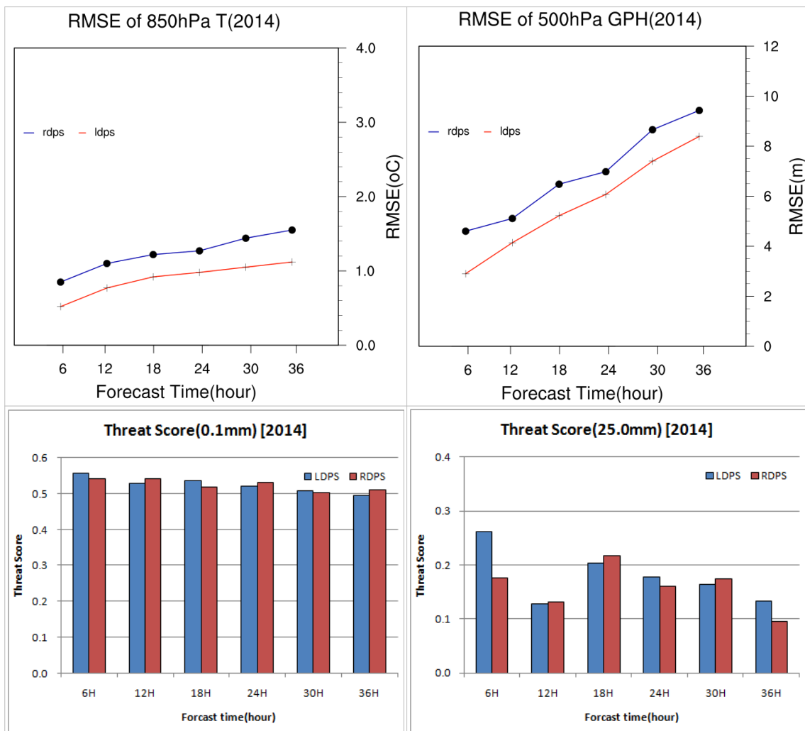
그림 2.10 지역예측시스템(UM 12km L70)과 국지예측시스템(LDAPS)의 2014년 분석검증 RMSE 및 강수 성공임계지수 비교
