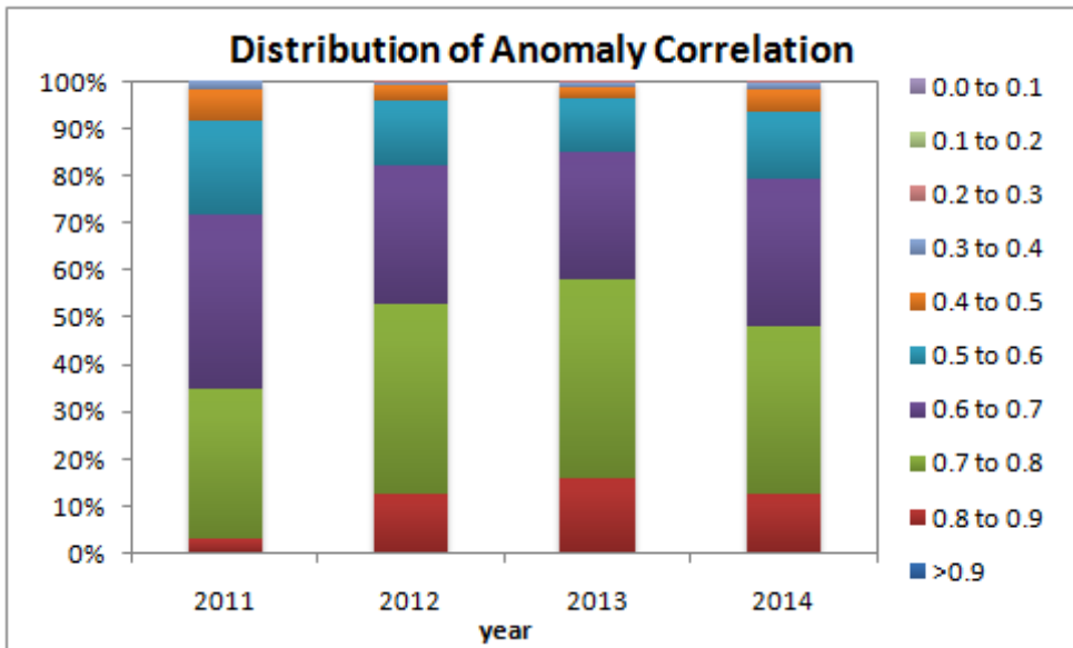
그림 2.6 전지구예측시스템(GDAPS) 7일 북반구 500hPa 고도 분석검증에 대한 이상상관 계수의 년별 분포(2011년의 경우 5월~12월)
