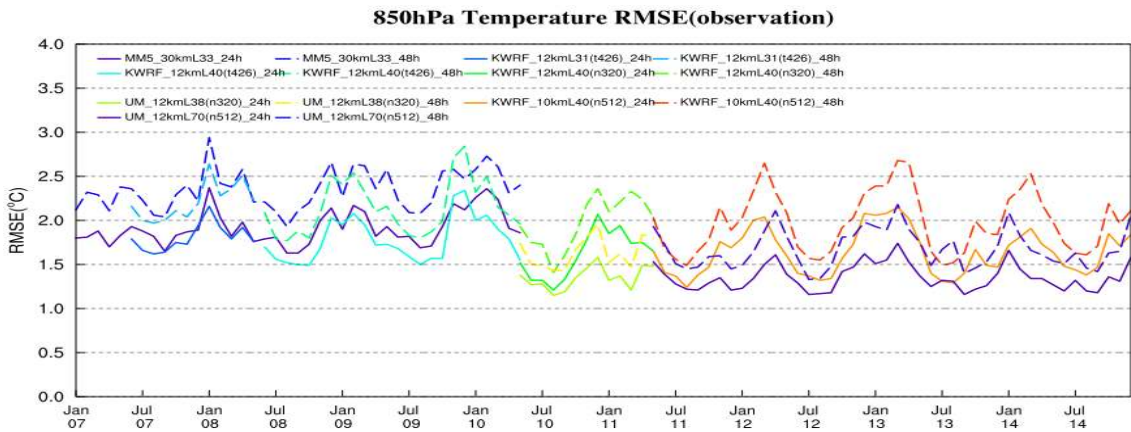
그림 3.2.5 RDAPS 850hPa 기온의 관측검증 RMSE의 월평균 시계열
