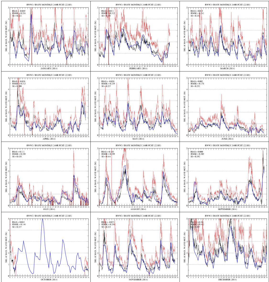
그림 3.6.14 동해 부이 관측(검은색 실선)과 RWW3 +24H 예측 유의파고(파란색 실선) 시계열 (2014년 1월~12월). 붉은색 점선은 최대 파고
