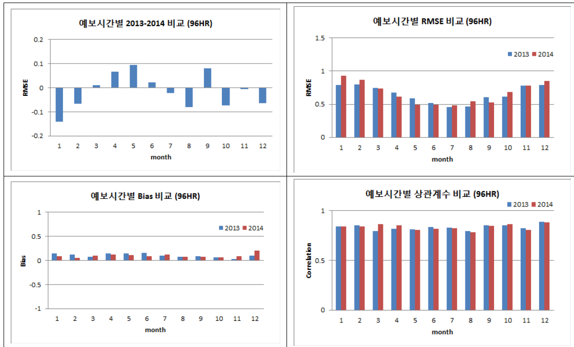
그림 3.6.8 GWW3 +96H 예보장에 대한 전년 대비 성능 비교. BIAS, RMSE, Correlation
