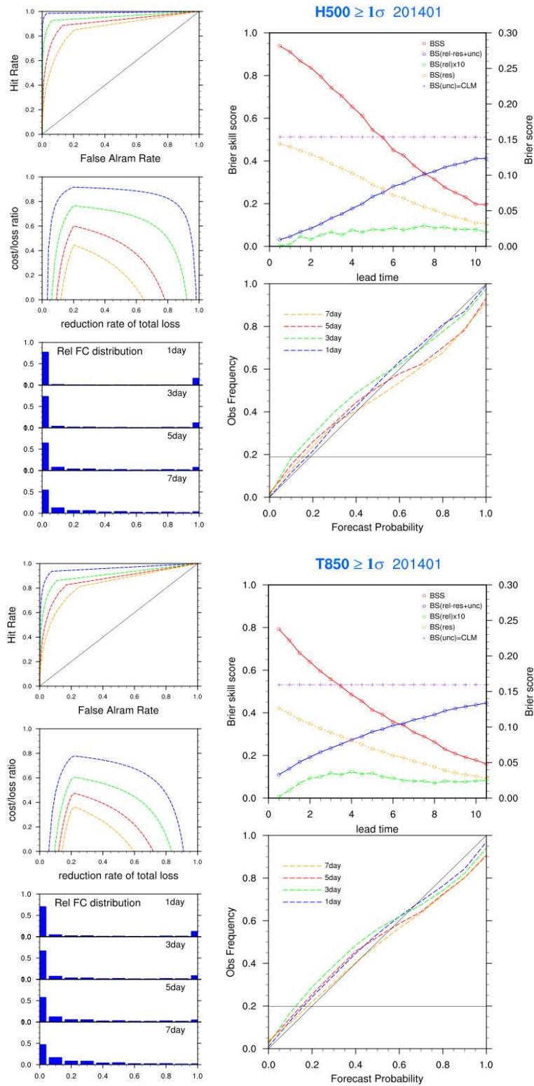
그림 3.4.7 2014년 1월 EPSG 북반구 500 hPa 고도(상)와 850hPa 기온(하)의 +1 표준편차에 대한 확률예측 성능 (왼쪽 상단부터 ROC curve, Economic Value, Rank histogram, 오른쪽 상단부터 Brier Score, Reliability Table)
