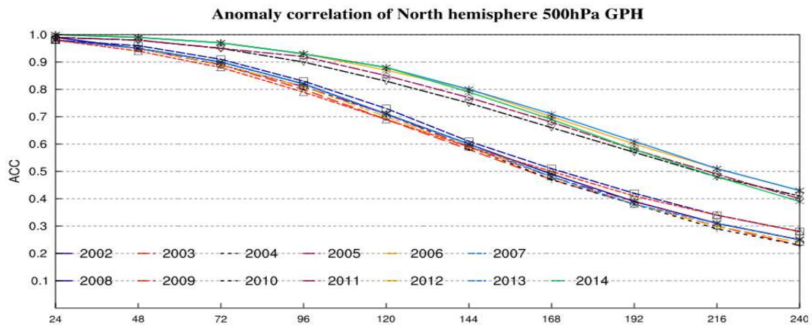
그림 2.4 전지구예측시스템(GDAPS) 북반구 500hPa 고도 분석검증 이상상관 계수 예보시간별, 년별 변화
