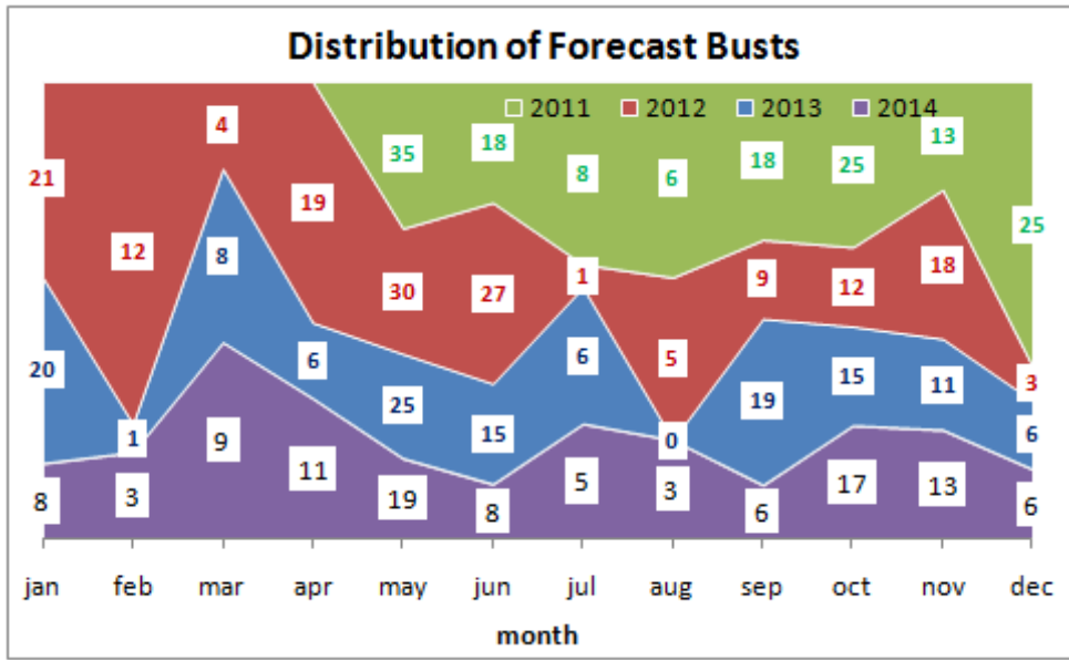
그림 2.5 전지구예측시스템(GDAPS) 5일 북반구 500hPa 고도 분석검증에 대한 forecast Bust의 년별 및 월별 분포(2011년의 경우 5월~12월)
