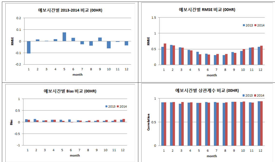
그림 3.6.4 GWW3 +00H 예보장에 대한 전년 대비 성능 비교. BIAS, RMSE, Correlation
