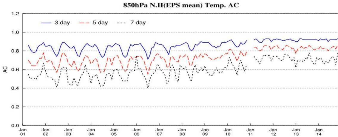
그림 3.4.5 EPSG 북반구 850hPa 기온의 예측 시간별 월평균 이상상관 계수
