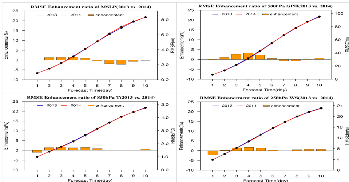
그림 2.1 전지구예측시스템(GDAPS) 북반구 분석검증 RMSE 2013년 대비 2014년 개선 정도
