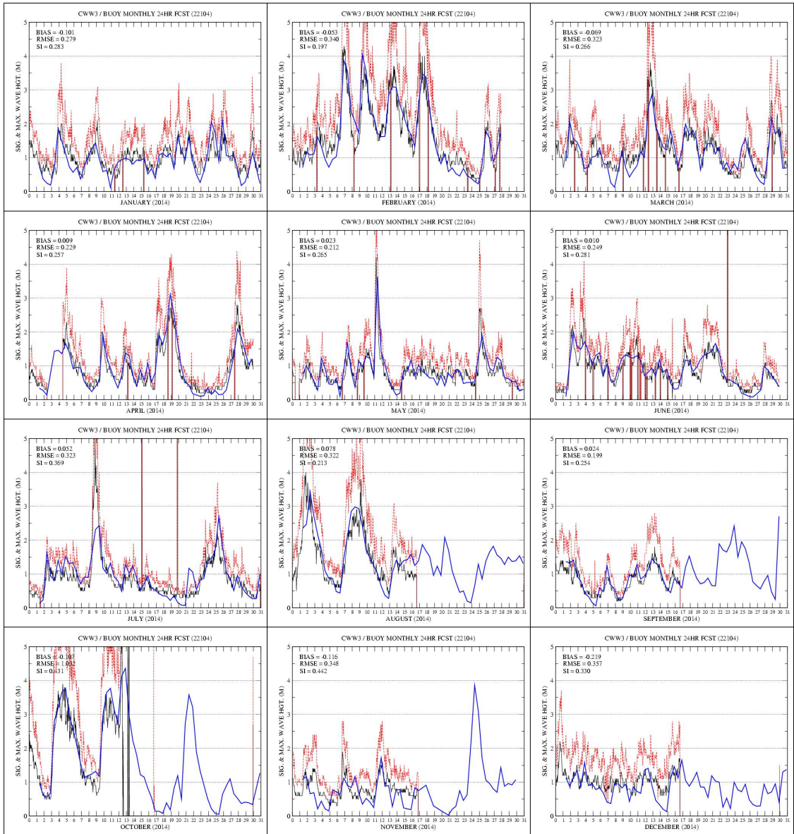
그림 3.6.21 거제도 부이 관측(검은색 실선)과 CWW3 +24H 예측 유의파고(파란색 실선) 시계열 (2014년 1월~12월). 붉은색 점선은 최대 파고
