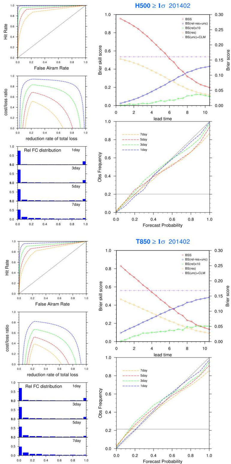
그림 3.4.8 2014년 2월 EPSG 북반구 500 hPa 고도(상)와 850hPa 기온(하)의 +1 표준편차에 대한 확률예측 성능 (왼쪽 상단부터 ROC curve, Economic Value, Rank histogram, 오른쪽 상단부터 Brier Score, Reliability Table)
