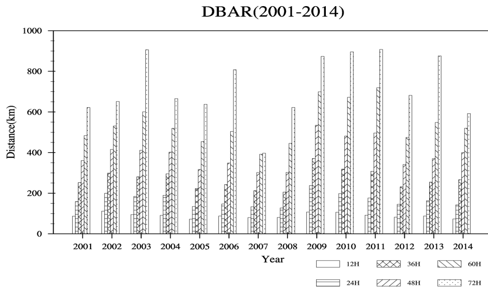
그림 3.7.4 현업태풍예측시스템(DBAR)의 태풍진로오차 성능 변화(2001~2003년(BATS), 2004~2014년(DBAR))
