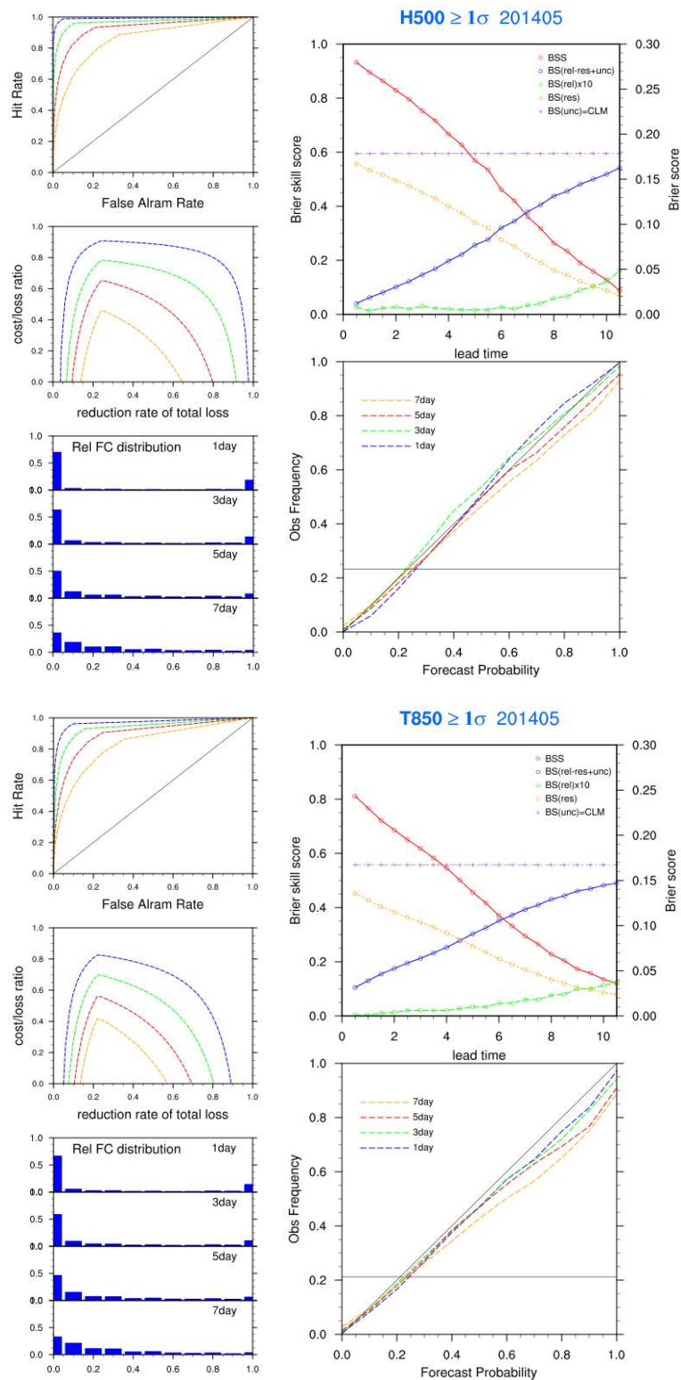
그림 3.4.11 2014년 5월 EPSG 북반구 500 hPa 고도(상)와 850hPa 기온(하)의 +1 표준편차에 대한 확률예측 성능 (왼쪽 상단부터 ROC curve, Economic Value, Rank histogram, 오른쪽 상단부터 Brier Score, Reliability Table)
