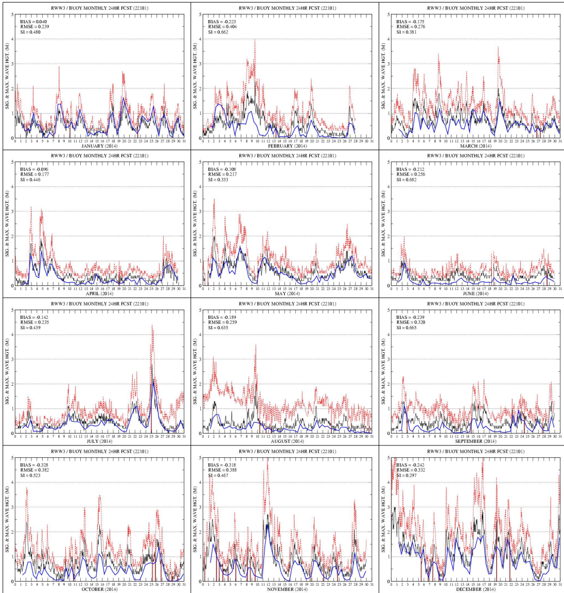
그림 3.6.10 덕적도 부이 관측(검은색 실선)과 RWW3 +24H 예측 유의파고(파란색 실선) 시계열 (2014년 1월~12월). 붉은색 점선은 최대 파고
