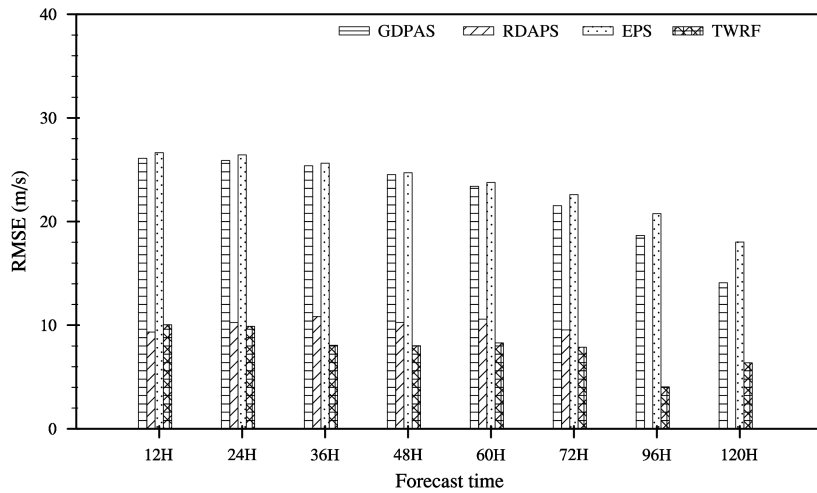
그림 3.7.14 2014년 모델별 태풍 최대풍속 평균제곱근오차(Root Mean Square Error)
