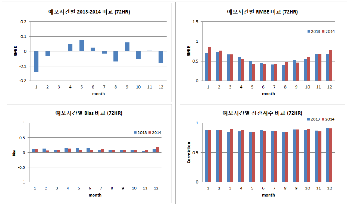
그림 3.6.7 GWW3 +72H 예보장에 대한 전년 대비 성능 비교. BIAS, RMSE, Correlation
