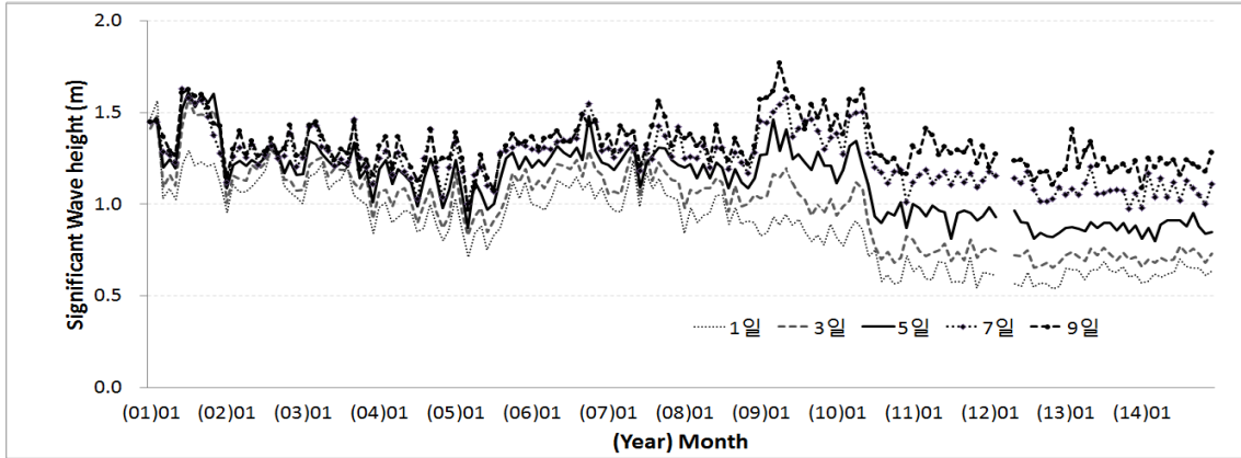
그림 3.6.1 전지구 파랑예측시스템(GWW3) 유의파고 위성검증 RMSE
