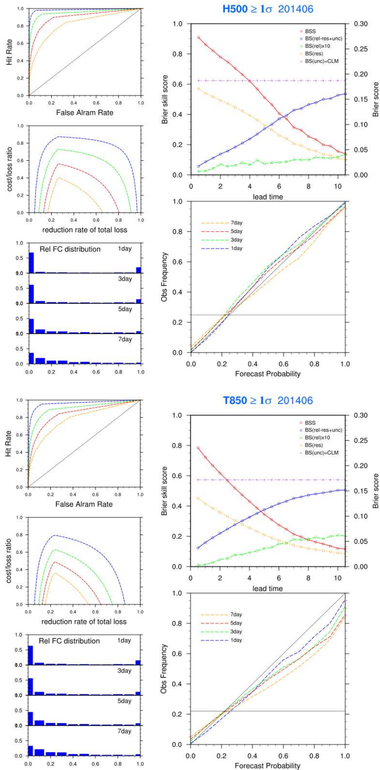
그림 3.4.12 2014년 6월 EPSG 북반구 500 hPa 고도(상)와 850hPa 기온(하)의 +1 표준편차에 대한 확률예측 성능 (왼쪽 상단부터 ROC curve, Economic Value, Rank histogram, 오른쪽 상단부터 Brier Score, Reliability Table)
