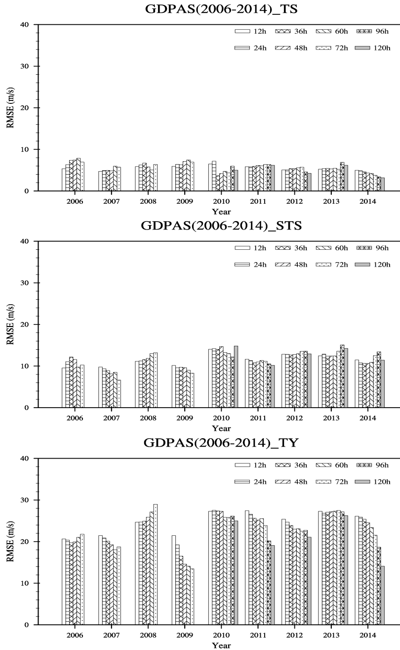
그림 3.7.10 전지구예측시스템(GDAPS)의 태풍 최대풍속 모의 성능 변화(2006~2009년 (T426L40), 2010년(UM N320L50), 2011년 이후(UM N512L70))
