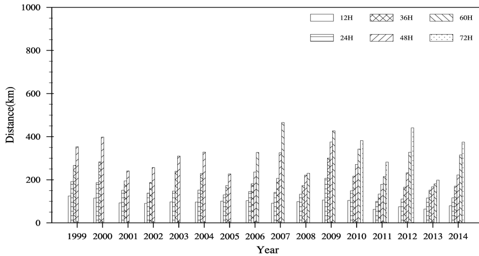
그림 3.7.2 지역예측시스템(RDAPS)의 태풍진로오차 성능 변화(2009년 이전(MM5 30km), 2010년 (UM 12km L38), 2011년 이후(UM 12km L70))
