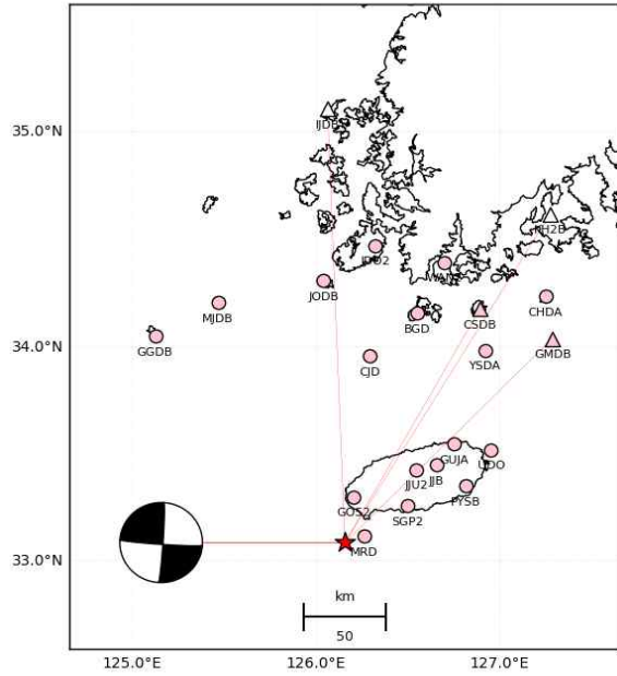
지진분석관측소 분포도
