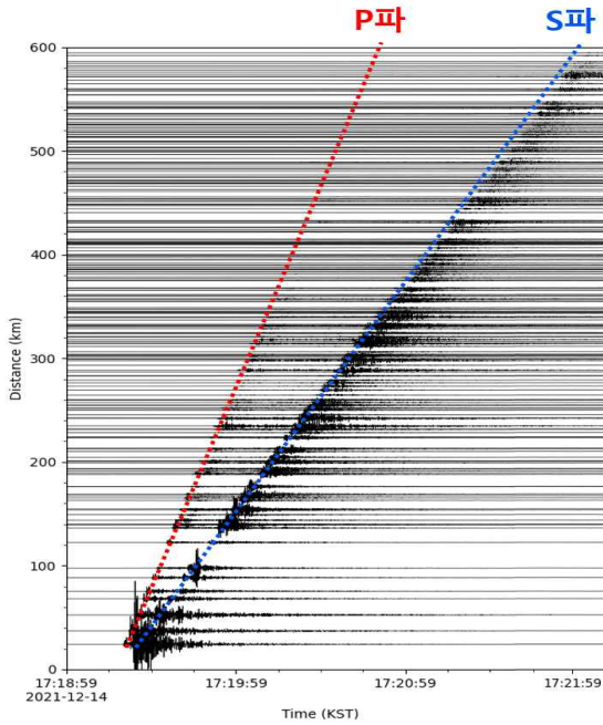
관측소 지진파형
