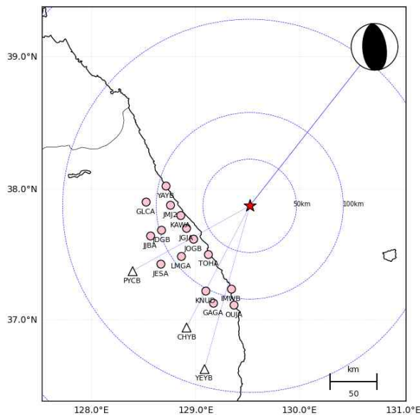
지진분석관측소 분포도
