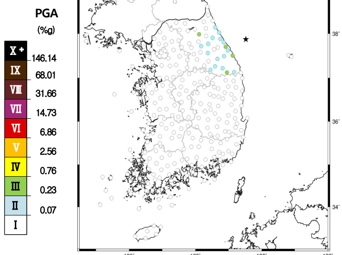
최대지반가속도 분포도
