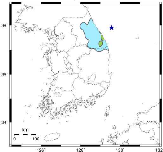
진도분포도
