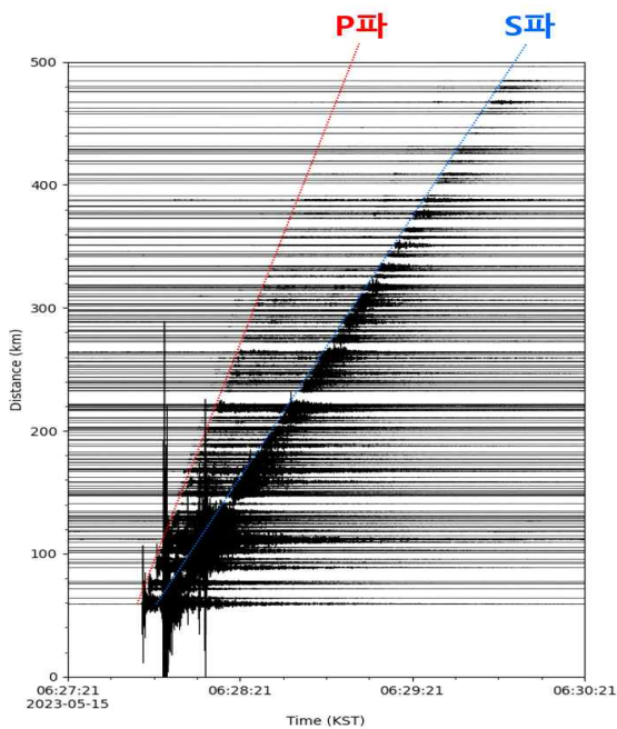
관측소 지진파형
