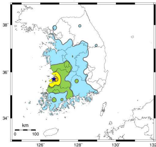
진도분포도
