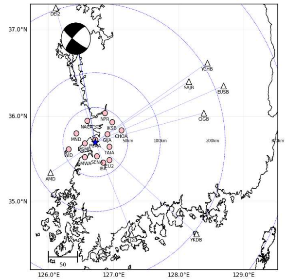
지진분석관측소 분포도
