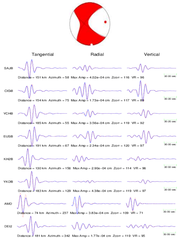
단층운동 분석결과
