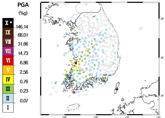
최대지반가속도 분포도
